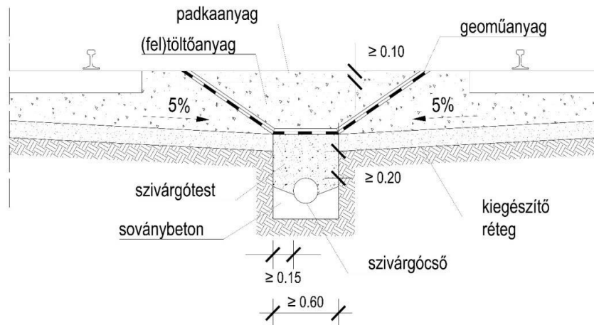
3. ábra: A felépítményi szivárgó elrendezése
