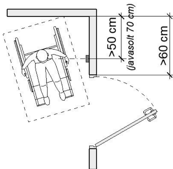
12. ábra: Példa ajtónyitó gomb elhelyezésére, ha az ajtó zárszerkezet felőli oldalán elegendő hely van a gomb eléréséhez
