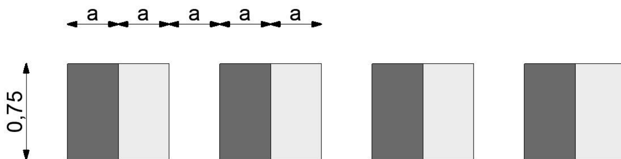
14. ábra: Példa üvegfelület jelzésére alkalmas jelsorra az MSZ EN 16584-1 szabvány szerint. A magasság 75 mm, az „a” méret legalább 30 mm. A jelek között átlátszó üvegfelületi mező van.
